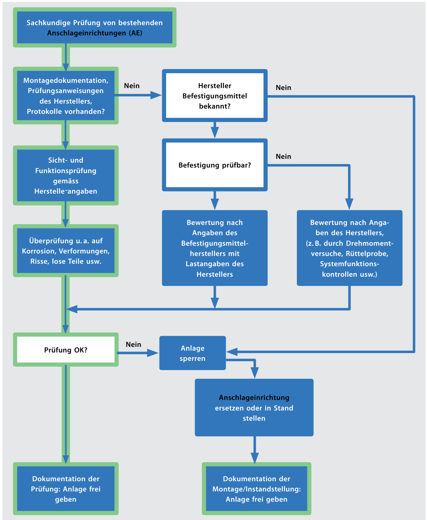
Abb. 45: Schema der jährlichen Prüfung einer Anschlagseinrichtung
