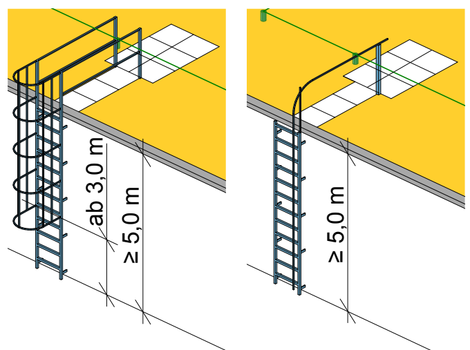
Abb. 38: Zugang über eine ortsfeste Leiter mit Rückenschutz oder Steigschutz (Steigschutz ist dem Rückenschutz vorzuziehen).
