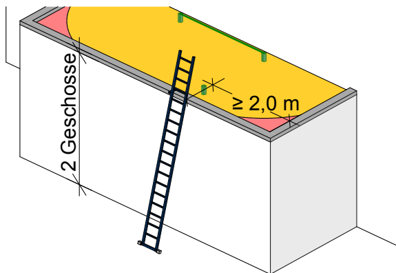
Abb. 36: Zugang über eine Anstellleiter nur bis zwei Geschosse (ca. 6 m) empfohlen.
