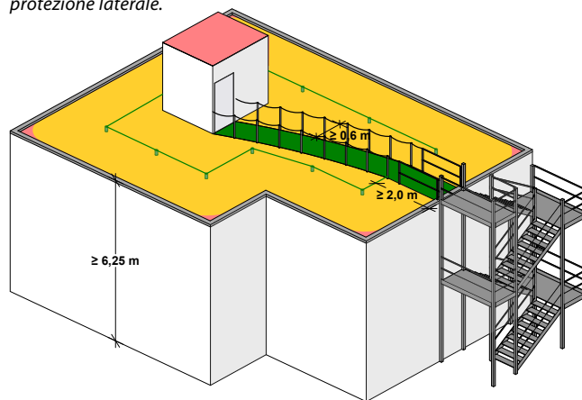
Fig. 21: Passerella o via di fuga, almeno doppio parapetto, almeno 2 m di guida rigida all'interno dell'area e successiva segnalazione del percorso con restrizione di zona (catena o corda)
