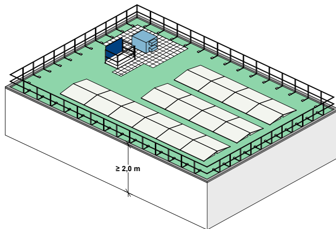
Fig. 22: Classe di allestimento 3: Protezione collettiva consigliata per i tetti piani che devono essere avviati più volte all'anno per la manutenzione o altri lavori.
