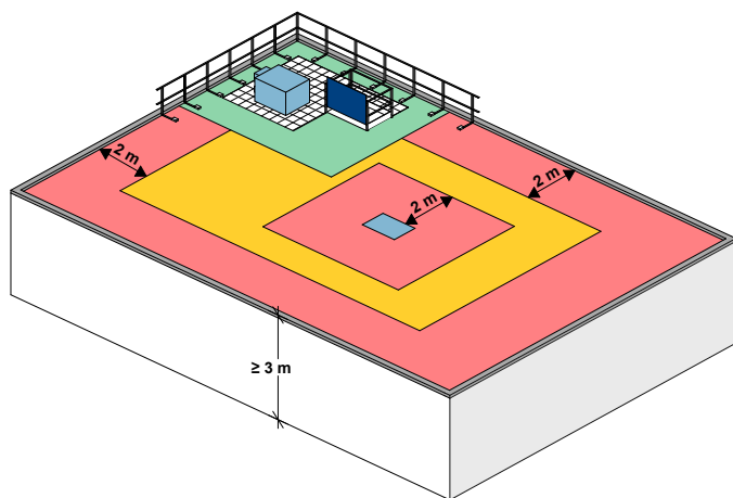
Fig. 2: (Verde) Area sicura non pubblica, (Giallo) Zona pericolosa interna, (Rosso) Zona pericolosa con alto rischio di caduta, (Azzurro chiaro) Elemento di luce diurna non a prova di sfondamento o apertura del tetto
