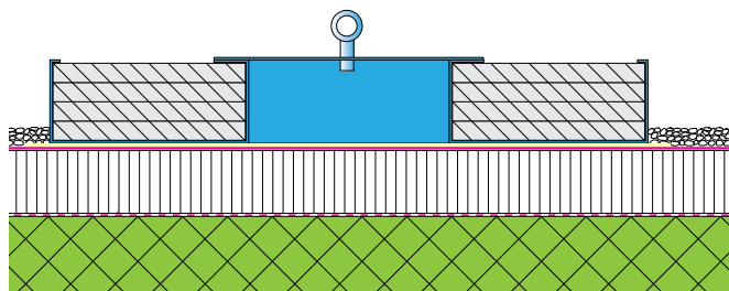
Fig. 7: Classe di allestimento 1: Dispositivi di ancoraggio mantenuti da zavorra, senza penetrazione dell'impermeabilizzazione (EN 795 tipo E). Questi punti possono essere utilizzati anche temporaneamente. Occorre verificare se sono omologati per lavori in condizioni di gelo, ad esempio per lo sgombero della neve. (Osservare le istruzioni del produttore, verificare la resistenza alla compressione dell'isolamento e la statica del tetto).
