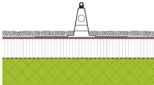
Fig. 6: Classe di allestimento 1; PAS installato su un tetto piano isolato termicamente, variante appesantita dal substrato sull'impermeabilizzazione. (Osservare le istruzioni del produttore, chiarire l'idoneità all'inverno).
