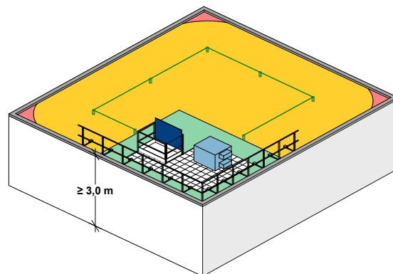
Fig. 20: Esempio di edificio industriale con unità di condizionamento sul tetto. Nel caso di impianti di ventilazione con manutenzione intensiva o con interventi che si protraggono per oltre due giorni per persona, queste superfici del tetto in classe di allestimento 3 devono essere dotate di una protezione laterale.
