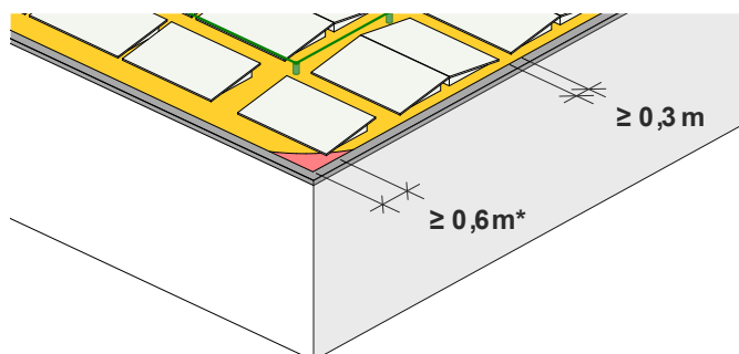
Fig. 27: Vie di circolazione min. 0,6 m
