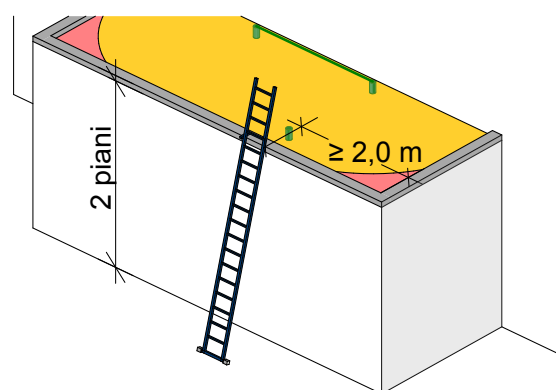
Fig. 37: L'accesso tramite una scala di accesso è consigliato solo fino a due piani (circa 6 m) per gli edifici di nuova progettazione.
