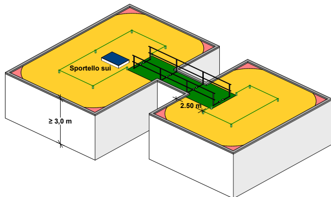
Fig. 18: Esempio di forme speciali del tetto. Installazione di apparecchi delle classi 2 e 3; nel passaggio verso l'altra zona del tetto, la fune dell'apparecchio della classe 2 non può essere installata a una distanza di 2,5 m, quindi si passa all'apparecchio della classe 3 con protezione laterale per questa zona.
