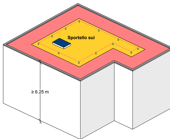
Fig. 13: Classe di allestimento 1: PAS sul bordo del tetto adattato alla geometria dell'edificio. L'ispezione viene effettuata con un sistema di cavi temporanei.
