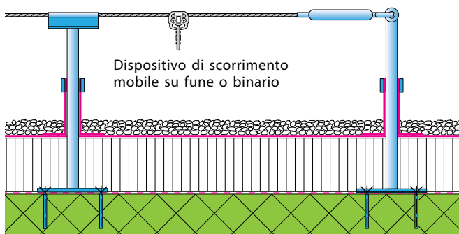
Fig. 14: Classe di allestimento 2: traino orizzontale permanente Sistema di cavi con dispositivo di tensionamento, ancorati direttamente
