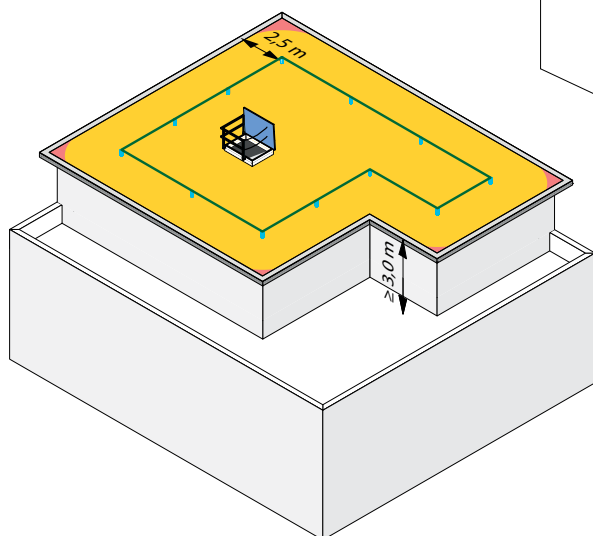
Fig. 15: Classe di allestimento 2: Utilizzare un sistema a fune o a binario se lo spazio libero di caduta è ridotto, ad esempio per terrazze in attico o edifici con spazio libero di caduta inferiore a 6,25 m.
