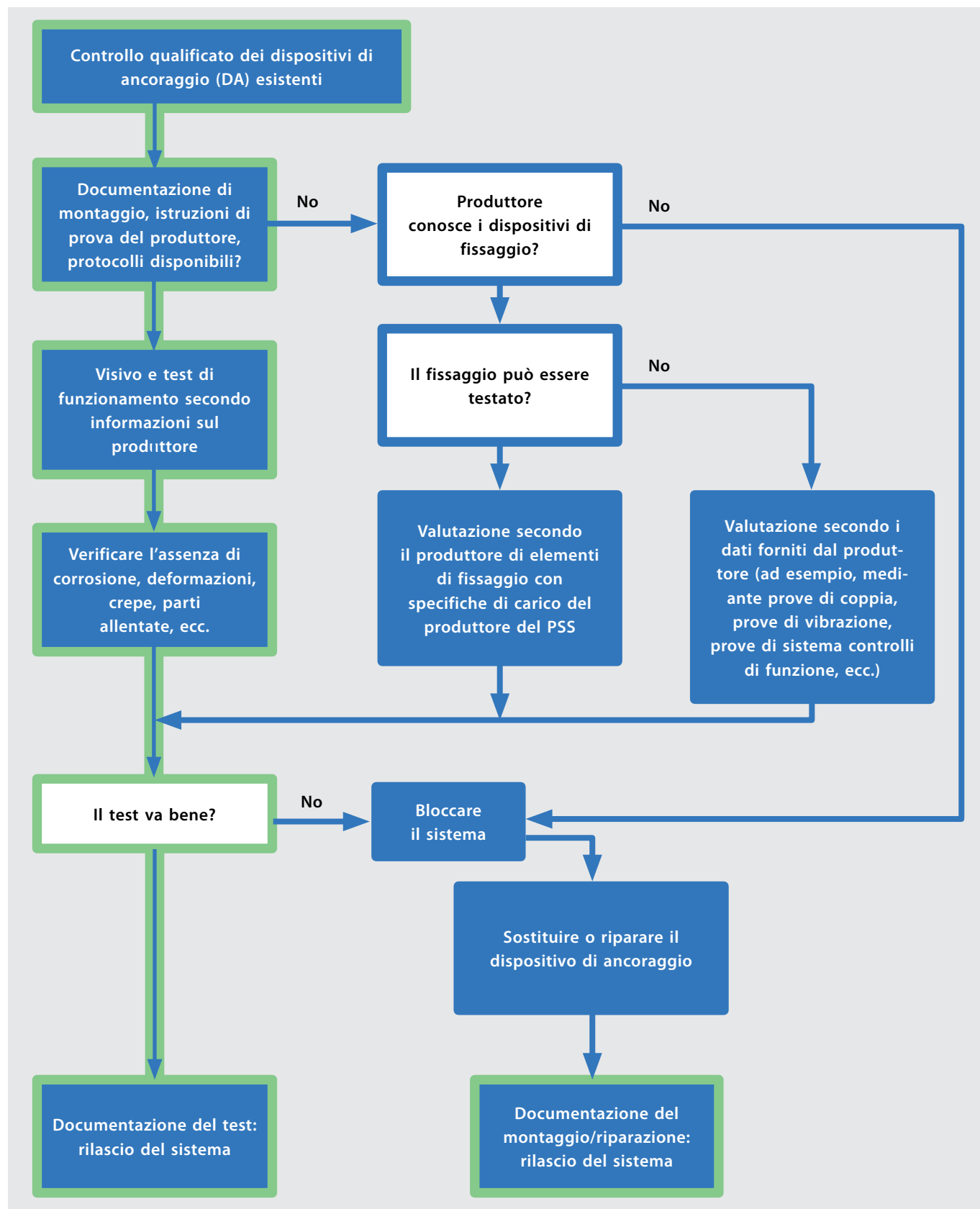
Fig. 46: Schema del controllo annuale di un dispositivo di ancoraggio
