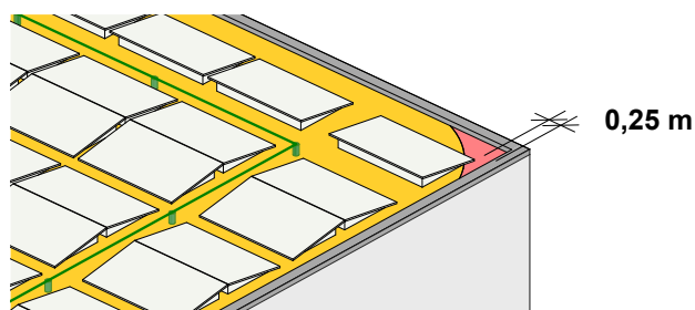
Fig. 28: Una distanza di 0,25 m consente in ogni caso un controllo del bordo del tetto, tuttavia questa zona non è praticabile.
