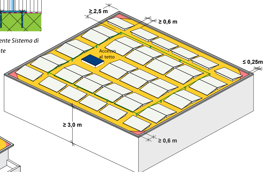
Fig. 16: Classe di allestimento 2: sistema di cavi installato in modo permanente per una superficie totale
