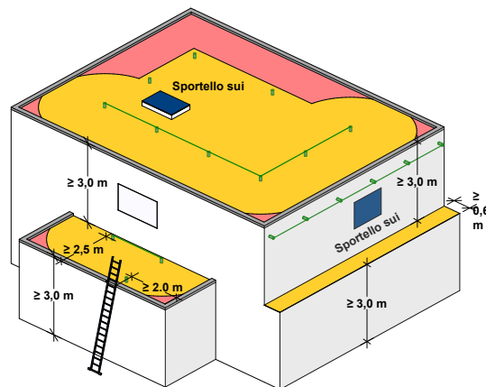
Fig. 19: Esempio di terrazza o edificio parapetto con estensione. Installazione di apparecchiature di classe 1 e 2. Se lo spazio di caduta è inferiore a 6,25 m, è necessario installare apparecchiature di classe 2 o utilizzare un cavo di sicurezza temporaneo. Se l'area da controllare ha una profondità inferiore a 2,5 m, è necessario adottare una misura adeguata, ad esempio un sistema di sicurezza sulla facciata.
