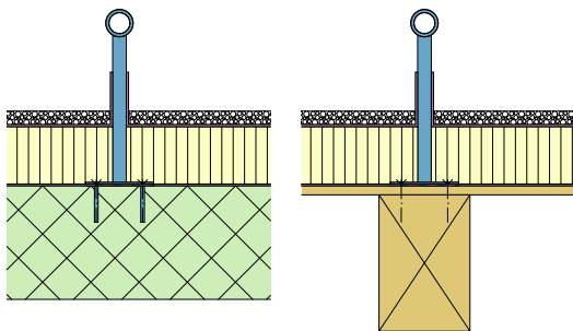
Fig. 5: Classe di allestimento 1: PAS installato su un tetto piano isolato termicamente, variante su una sottostruttura in calcestruzzo e legno
