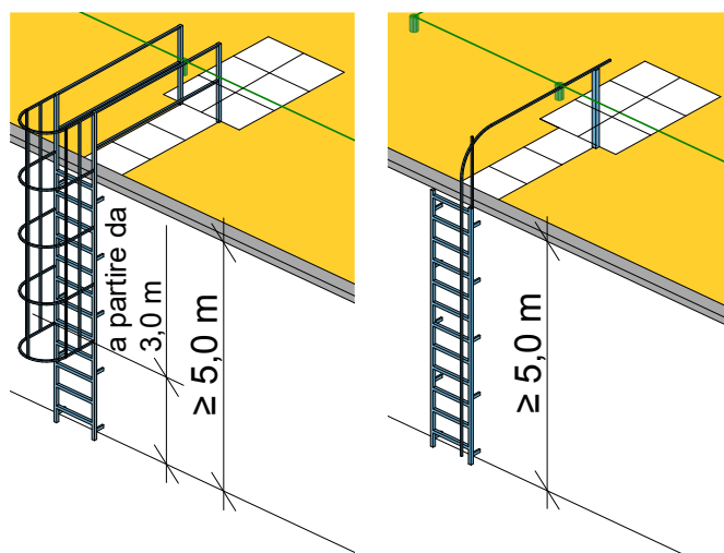
Fig. 39: Accesso tramite una scala fissa con protezione per la schiena o per l'arrampicata (la protezione per l'arrampicata è preferibile alla protezione per la schiena). L'installazione deve essere pianificata per il terreno.
